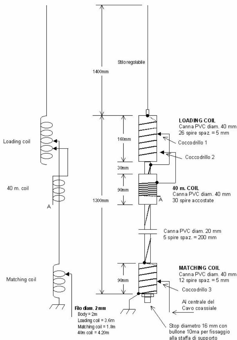
Figura 1 - Schema elettrico e costruttivo della verticale per HF
