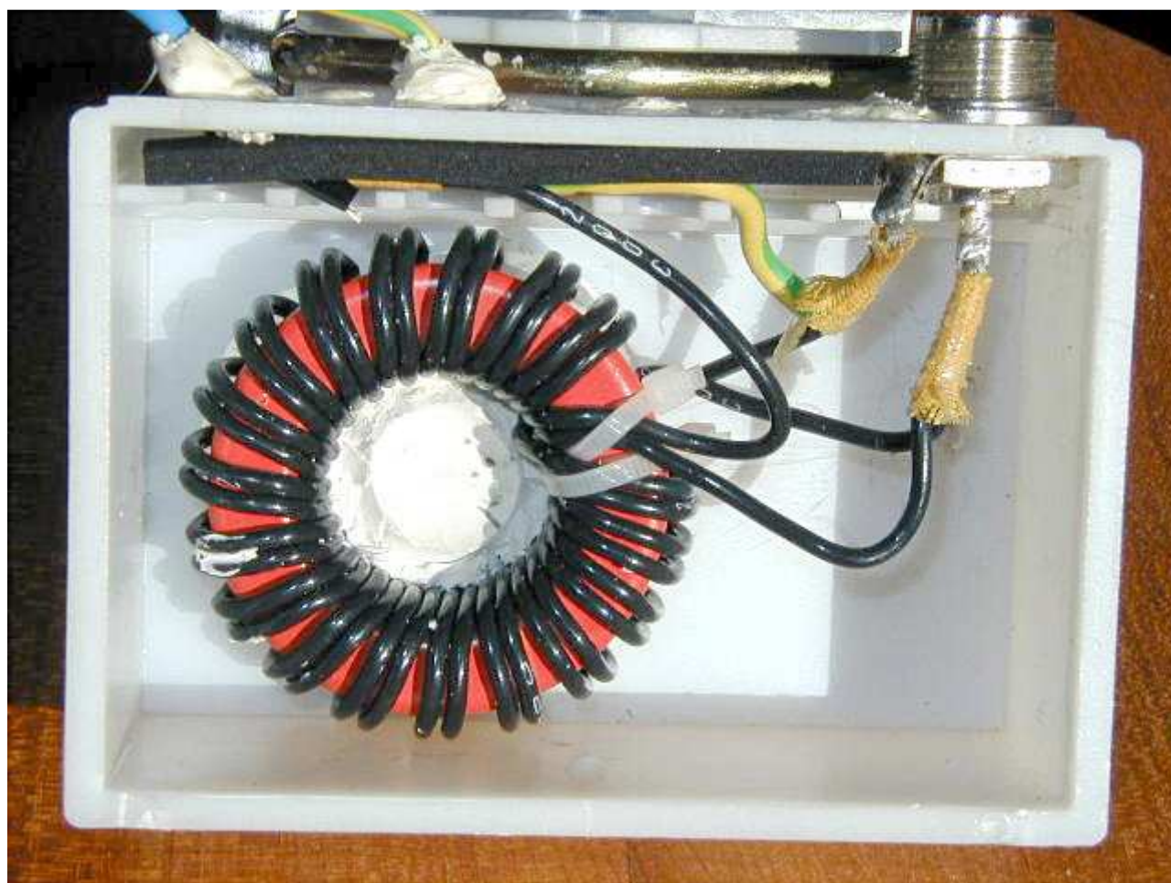
Primo piano dell'adattatore di impedenza 4:1
